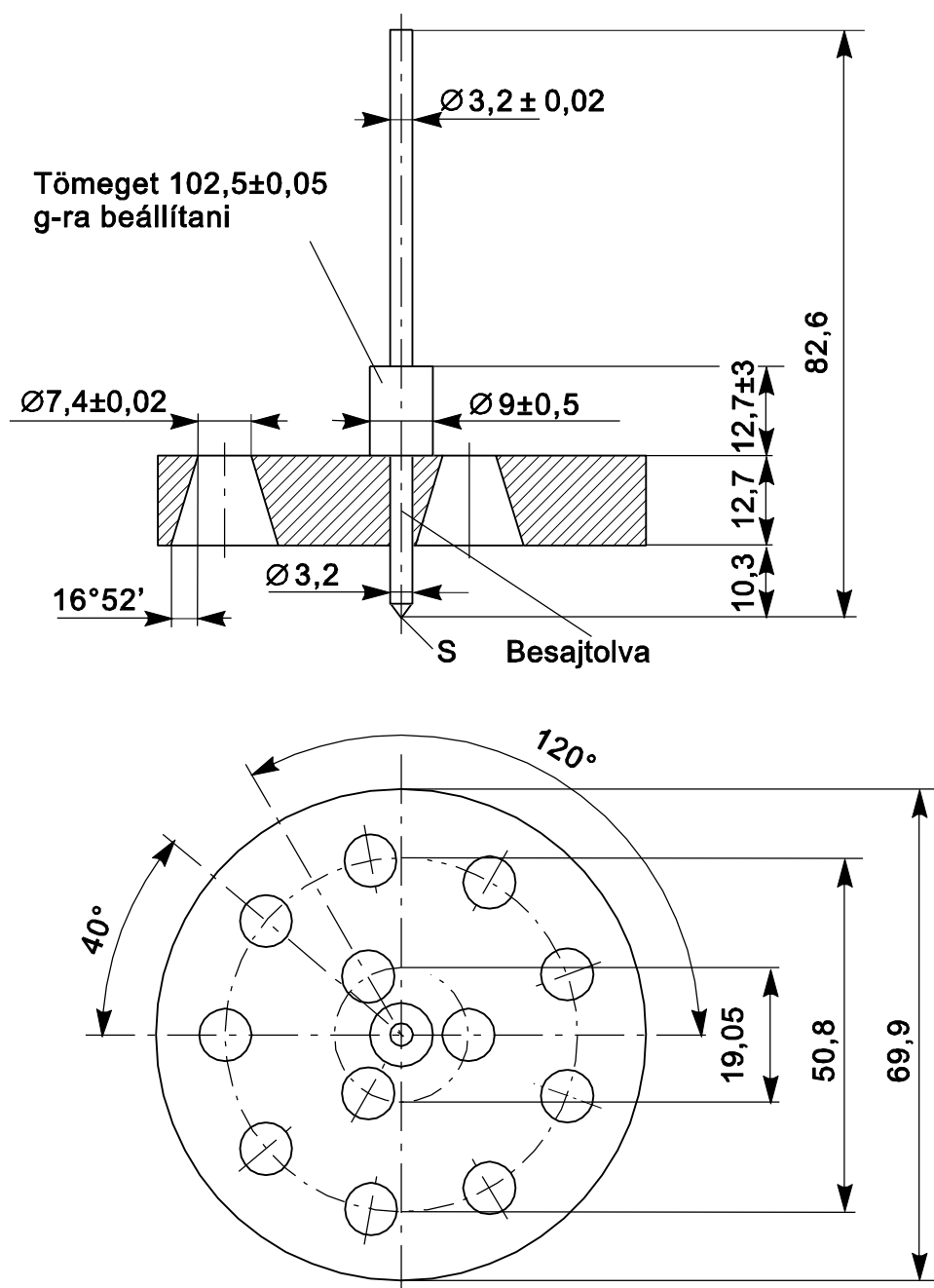
4. ábra: Penetrométer
