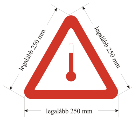
Magas hőmérsékleten szállított anyag jelölése
