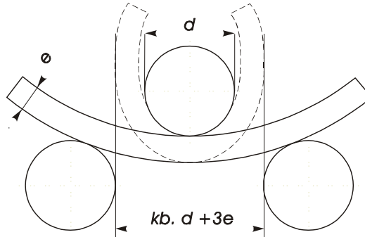
A hajlítási próba vázlata
